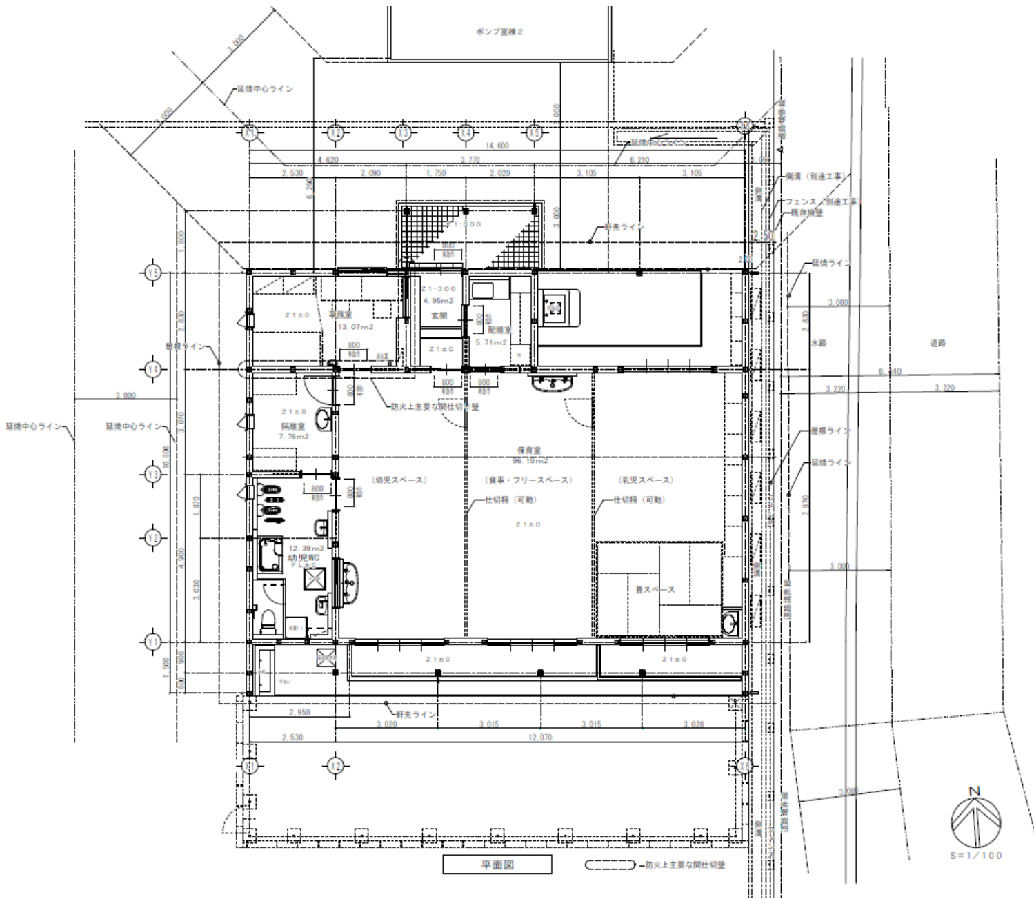
院内保育所平面图
